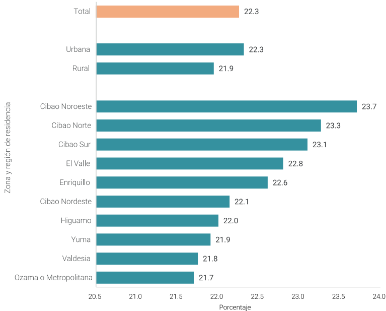
Promedio de horas al día que los hogares reciben el servicio de energía eléctrica, según zona de residencia y región de residencia
